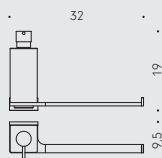
B1674 Spandisapone (L 0,31) e porta salvietta per bidet destro Right soap dispenser and towel holder for bidet
